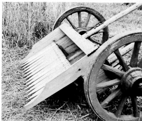
Reconstrucción contemporánea del vallus efectuado por ingenieros de la DLG alemana y un ensayo contemporáneo.
