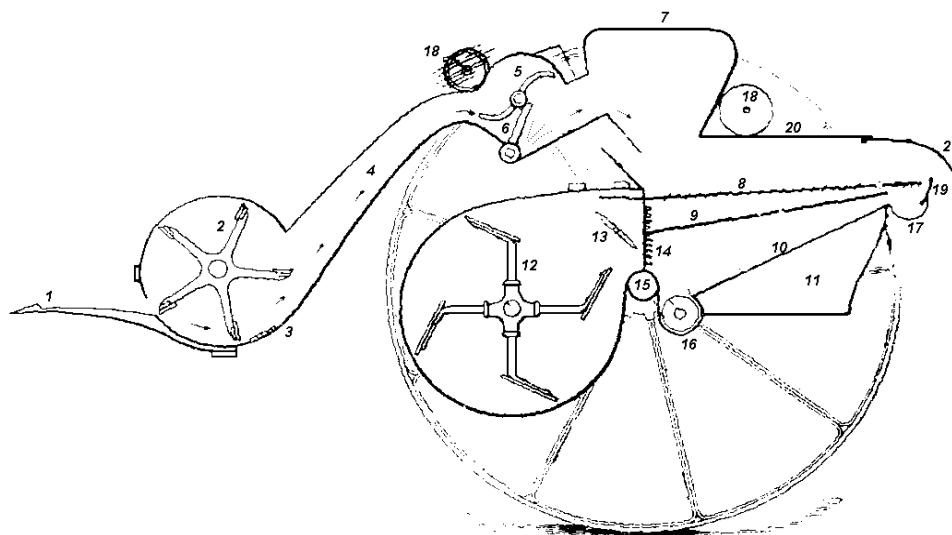
Corte esquemático de una "australiana"
